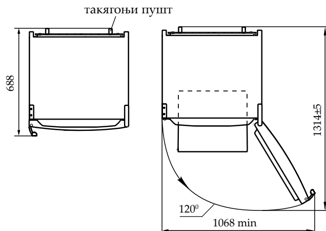
Расми 2 — Яхдон (нигоҳ аз боло)
