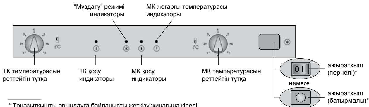
Сурет 5 — Басқару органдары және индикаторы
