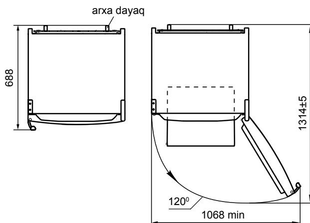
Şəkil 2 — Soyuducu (yuxarıdan görünüşü)
