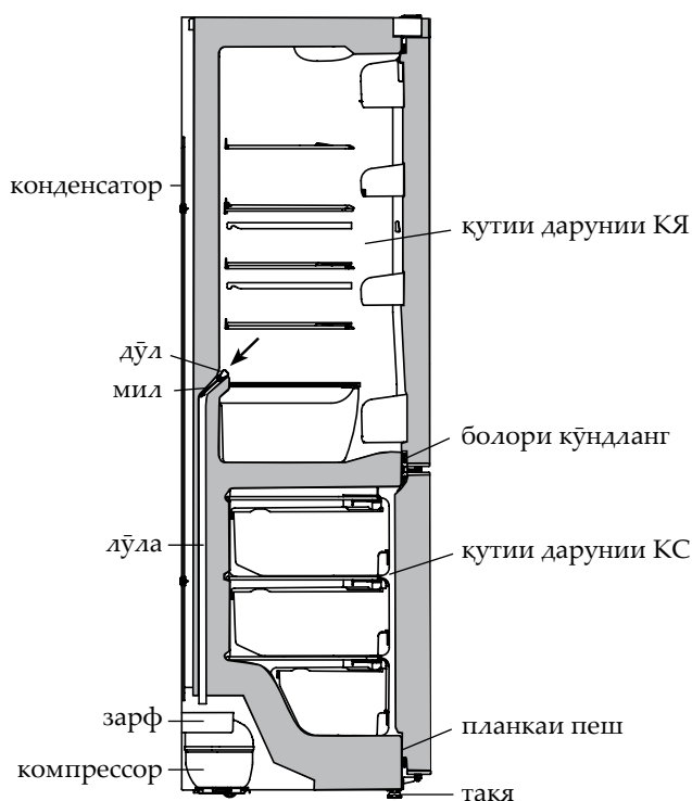
Расми 6 — Нақшаи партоби оби яхшуда аз КЯ
