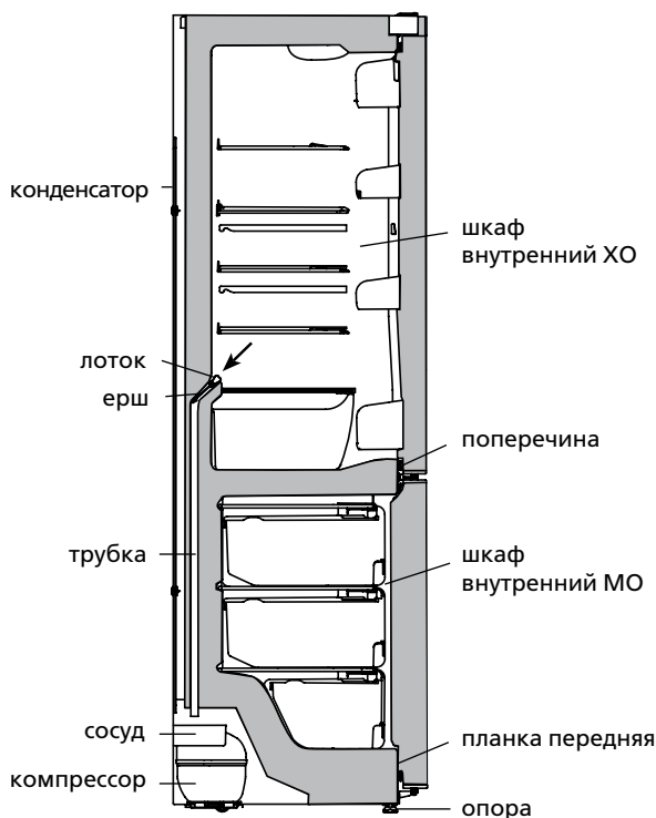
Рисунок 6 — Схема слива талой воды из ХО
