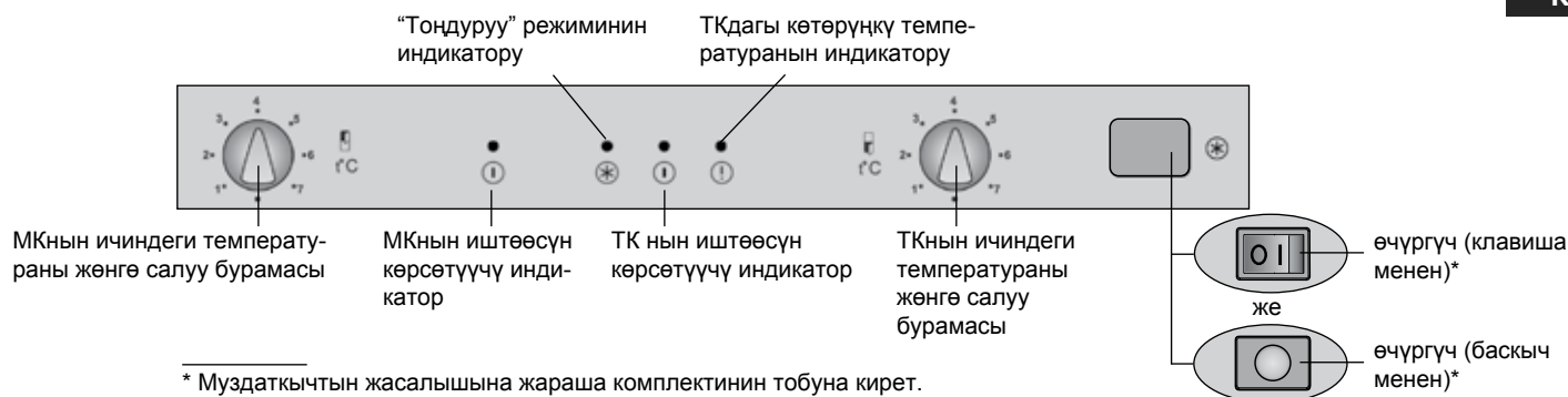
5-сүрөт – Индикациялоо жана башкаруу органдары
