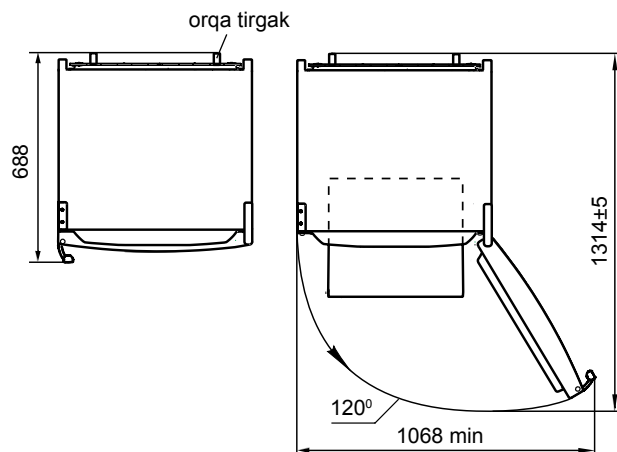
2-расм — Совутгич (тепадан кўриниши)
