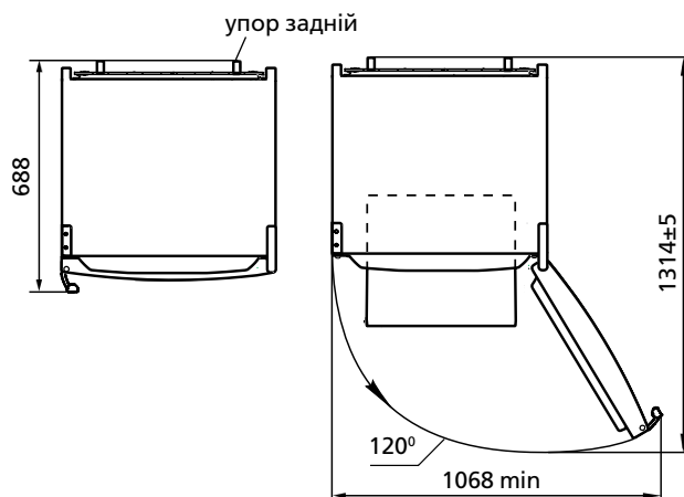
Рисунок 2 — Холодильник (вигляд зверху)
