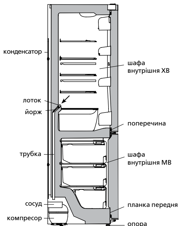
Рисунок 6 — Схема зливу талої води з ХВ
