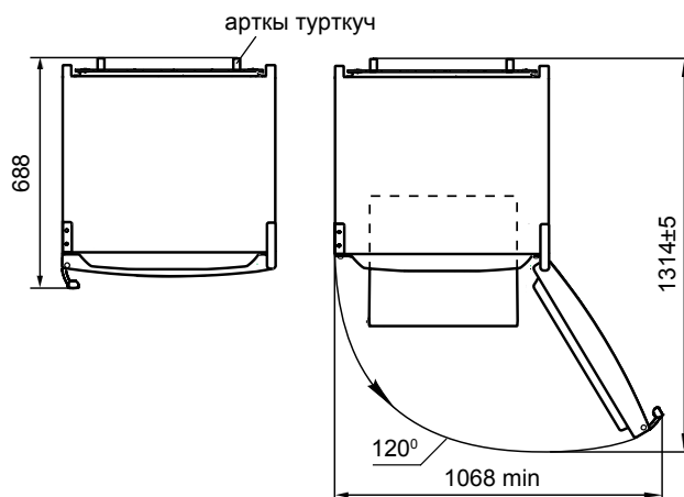
2-сүрөт – Муздаткыч (үстүнөн)
