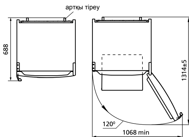
Сурет 2 — Тоңазытқыш (үстінен қарағанда)
