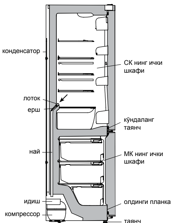
6-расм — СК дан эриган сувни тўкиш схемаси
