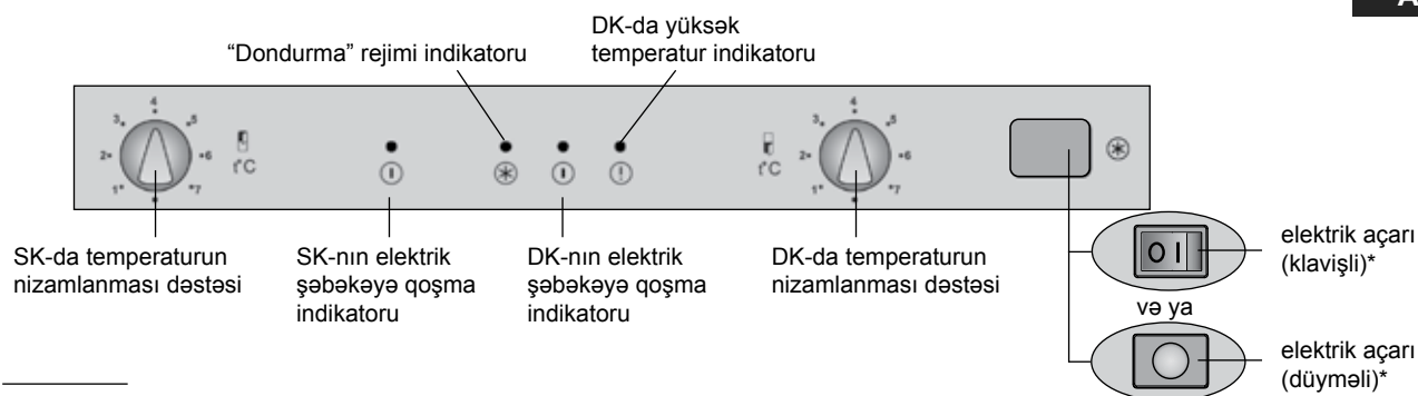
Şəkil 5 — İdarəetmə və indikasiya orqanları
