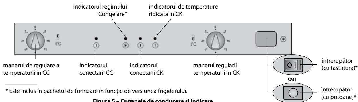
Figura 5 – Organele de conducere și indicare
