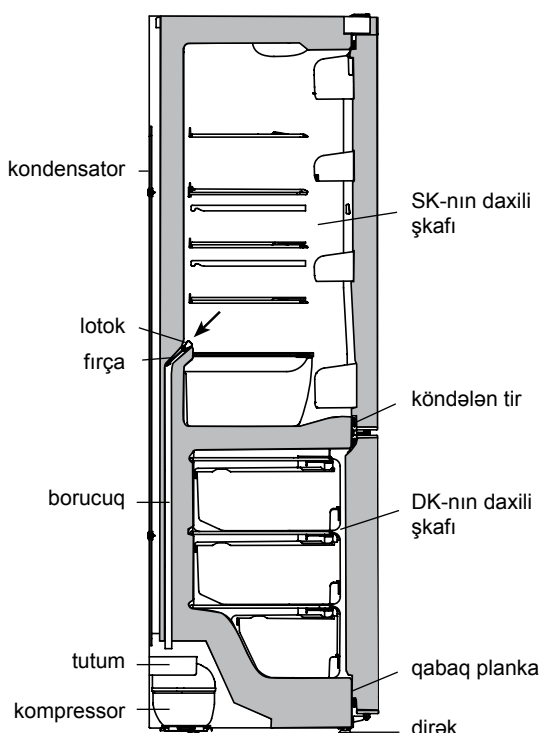
Şəkil 6 — Ərimiş suyun DK-dan axıdılması sxemi
