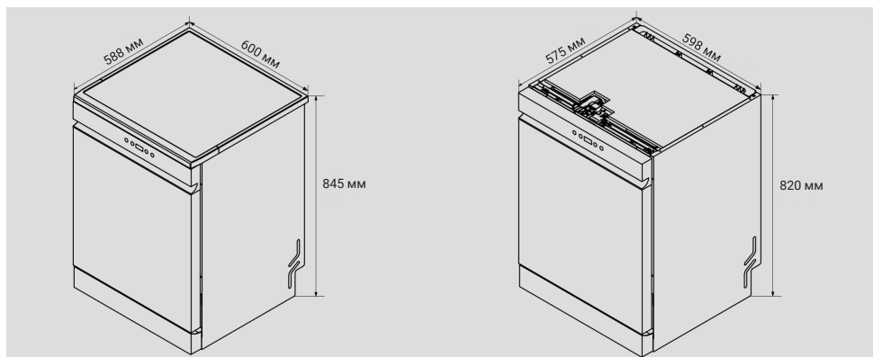
Размеры с установленной верхней крышкой
